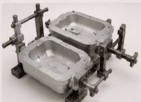
MOULAGE EN COQUILLE Coquille chauffée et assemblée.
