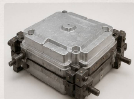
MOULAGE EN COQUILLE Coquille prête pour la coulée.
